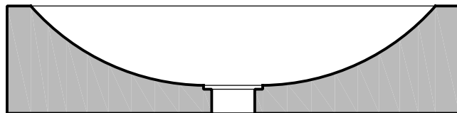
Sezione
