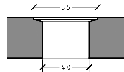
Sezione Scarico
