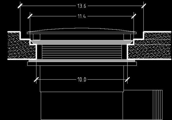
Sezione Scarico Piletta non inclusa
