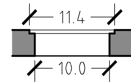
Sezione Scarico
