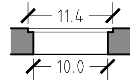
Sezione Scarico
