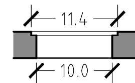
Sezione Scarico
