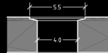
Sezione Scarico
