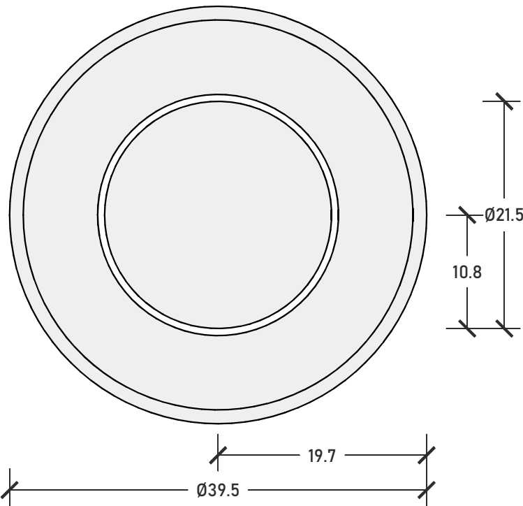
Pianta | Top
