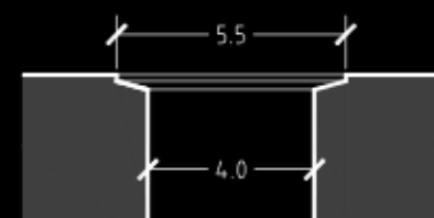
Sezione Scarico
