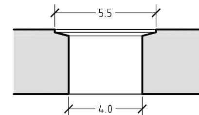
Sezione Scarico
